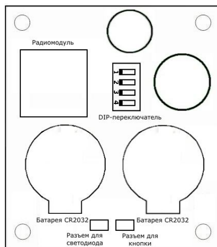
Рисунок 2. Внешний вид платы радиокнопки вызова MP-413W8
